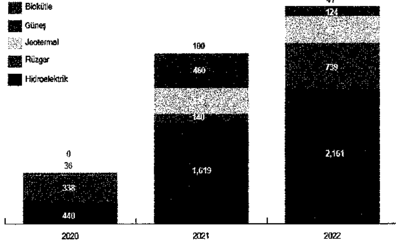
Kaynaklar Bazında Kurulu Güç (MW)
